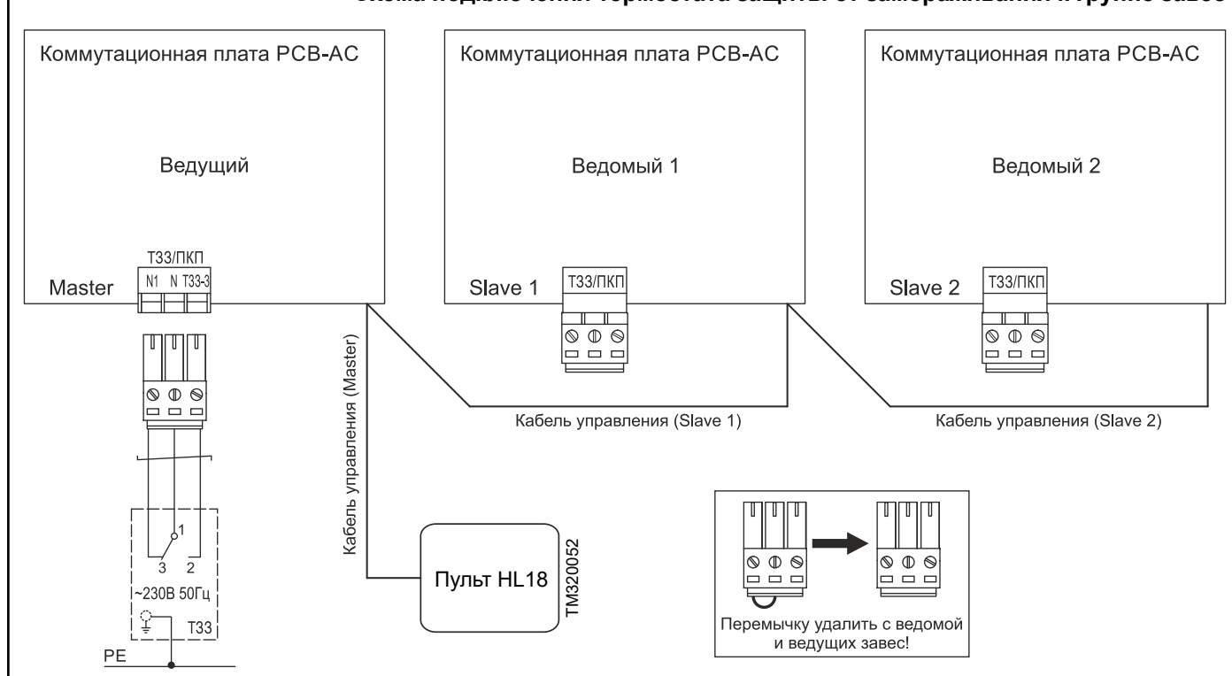
Схема подключения термостата защиты от замораживания к группе завес
