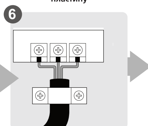
Подключите электропроводку
