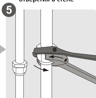
Соедините трубопроводы
