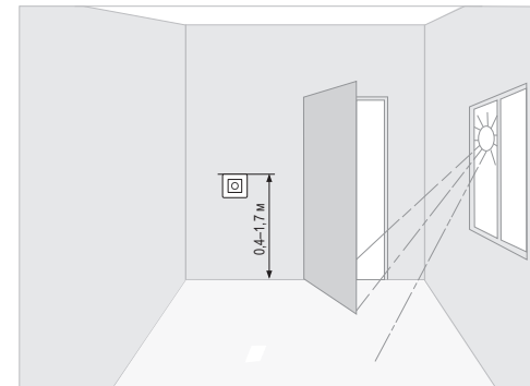
Рисунок 1. Монтаж терморегулятора
